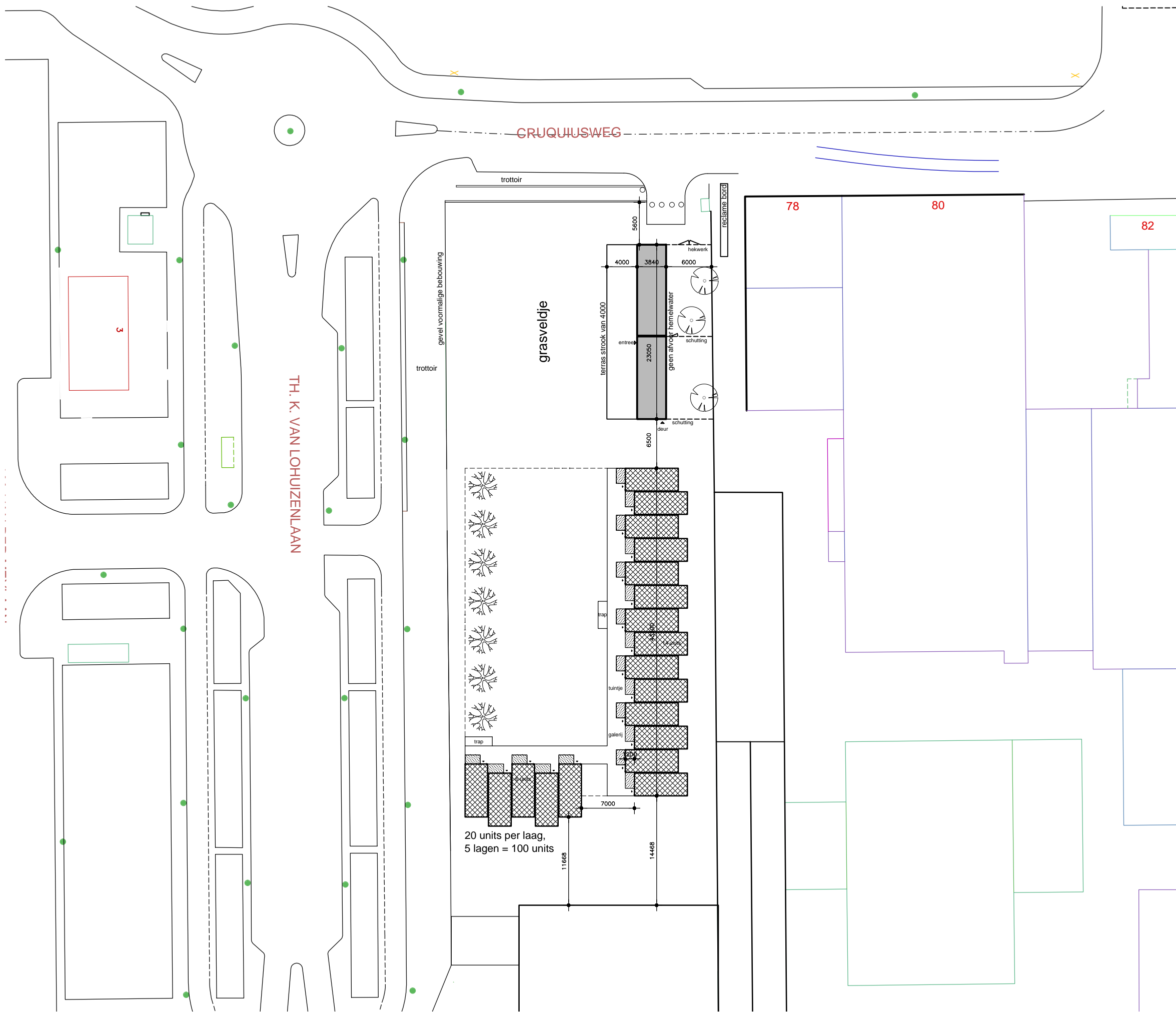
Plan B laag 1-5 schaal 1:500 d.d. 05-09-2016
