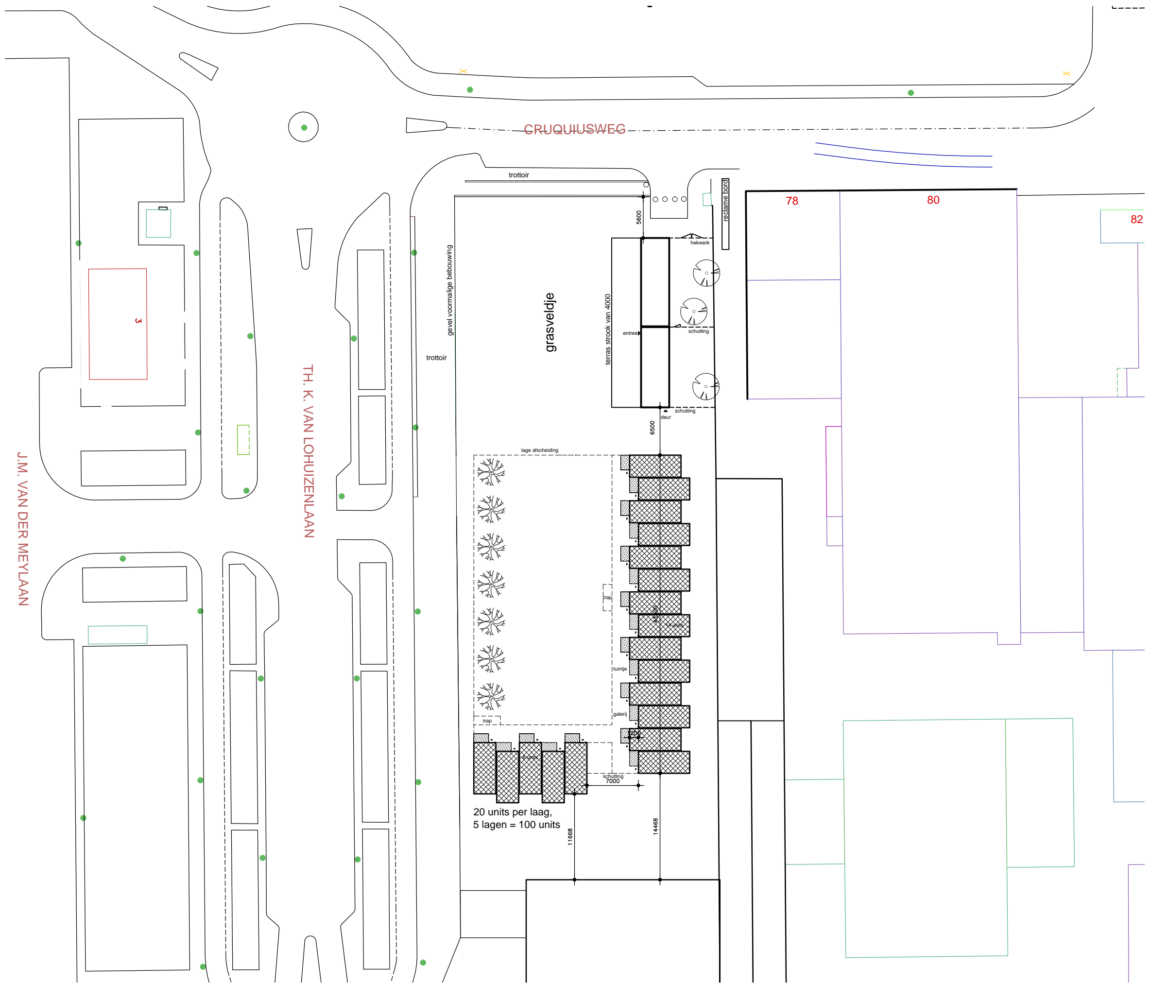
Plan B laag 0 schaal 1:500 d.d. 05-09-2016
